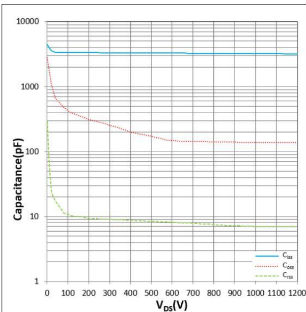
Figure 17. C_{iss} , C_{oss} , C_{rss} vs V_{DS} T_j = 25^\circ\text{C}
