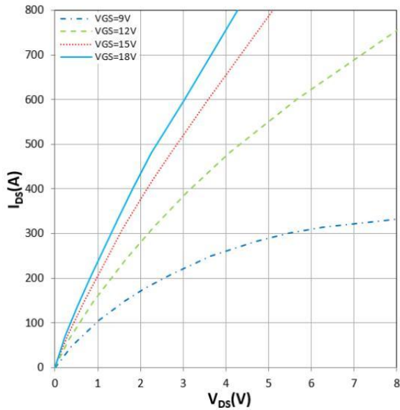
Figure 5. I_{DS} vs V_{DS}
